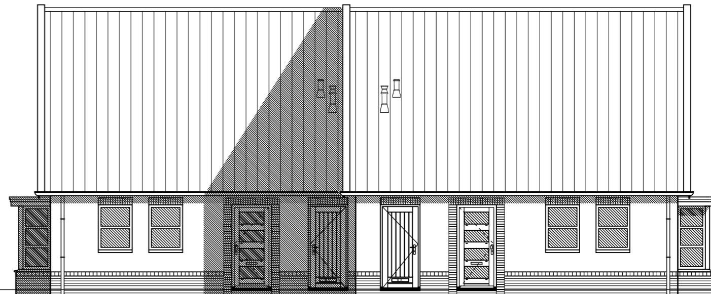
Voorgevel 4 P
