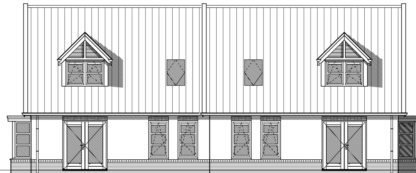
Achtergevel 4 P
