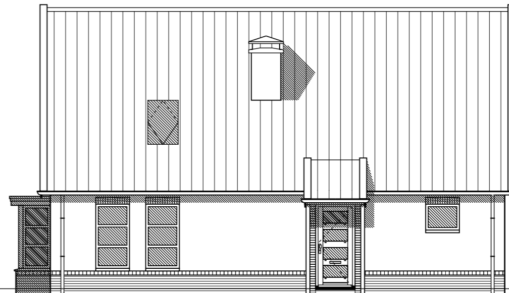
Voorgevel 8PL
