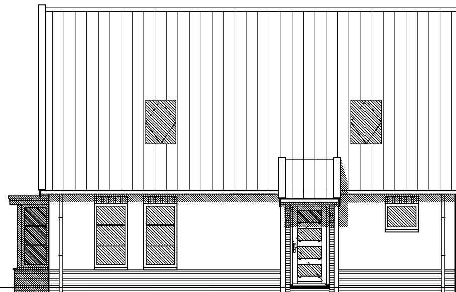
Voorgevel 8P
