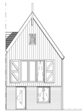
voorgevel
