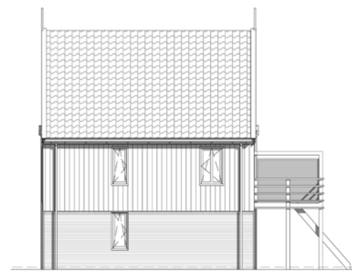
rechterzijgevel
