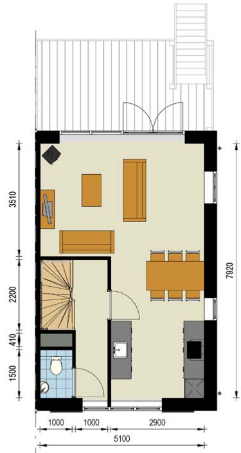
1e verdieping
