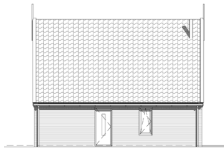
rechterzijgevel
