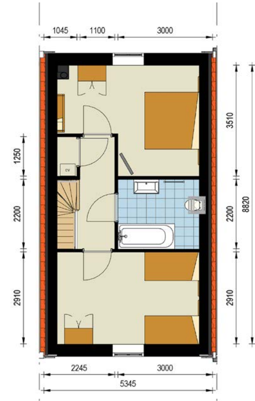
1e verdieping hoek- en tussenwoning
