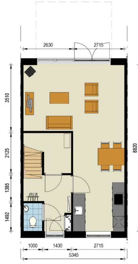
begane grond tussenwoning
