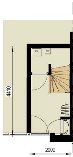
begane grond
