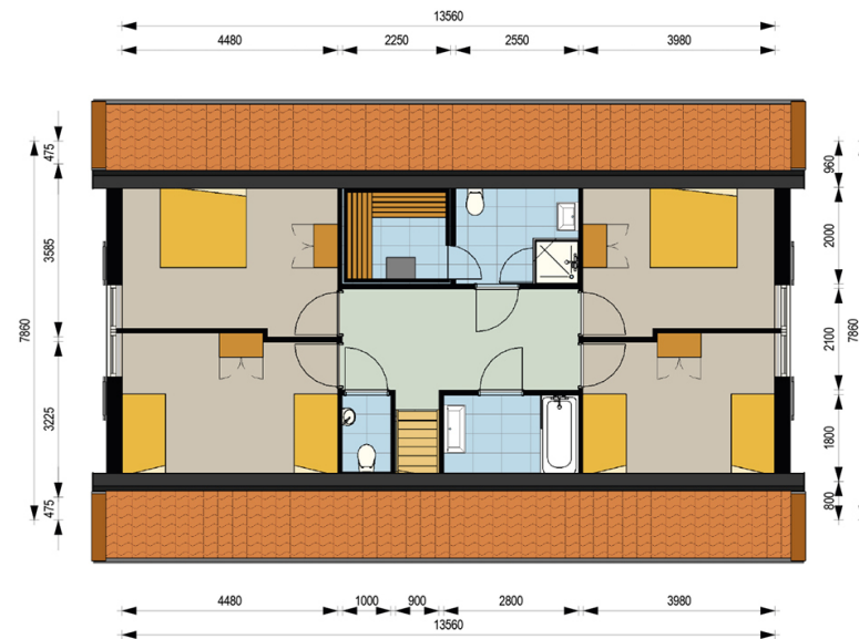
1e verdieping
