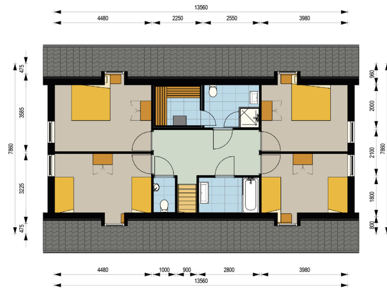
1e verdieping
