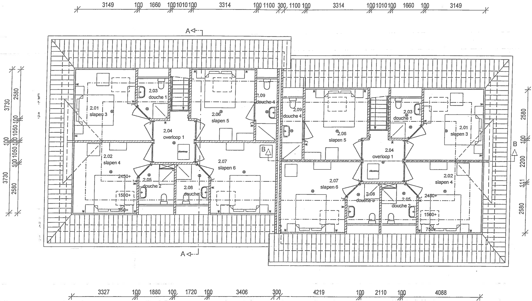
1e verdieping
