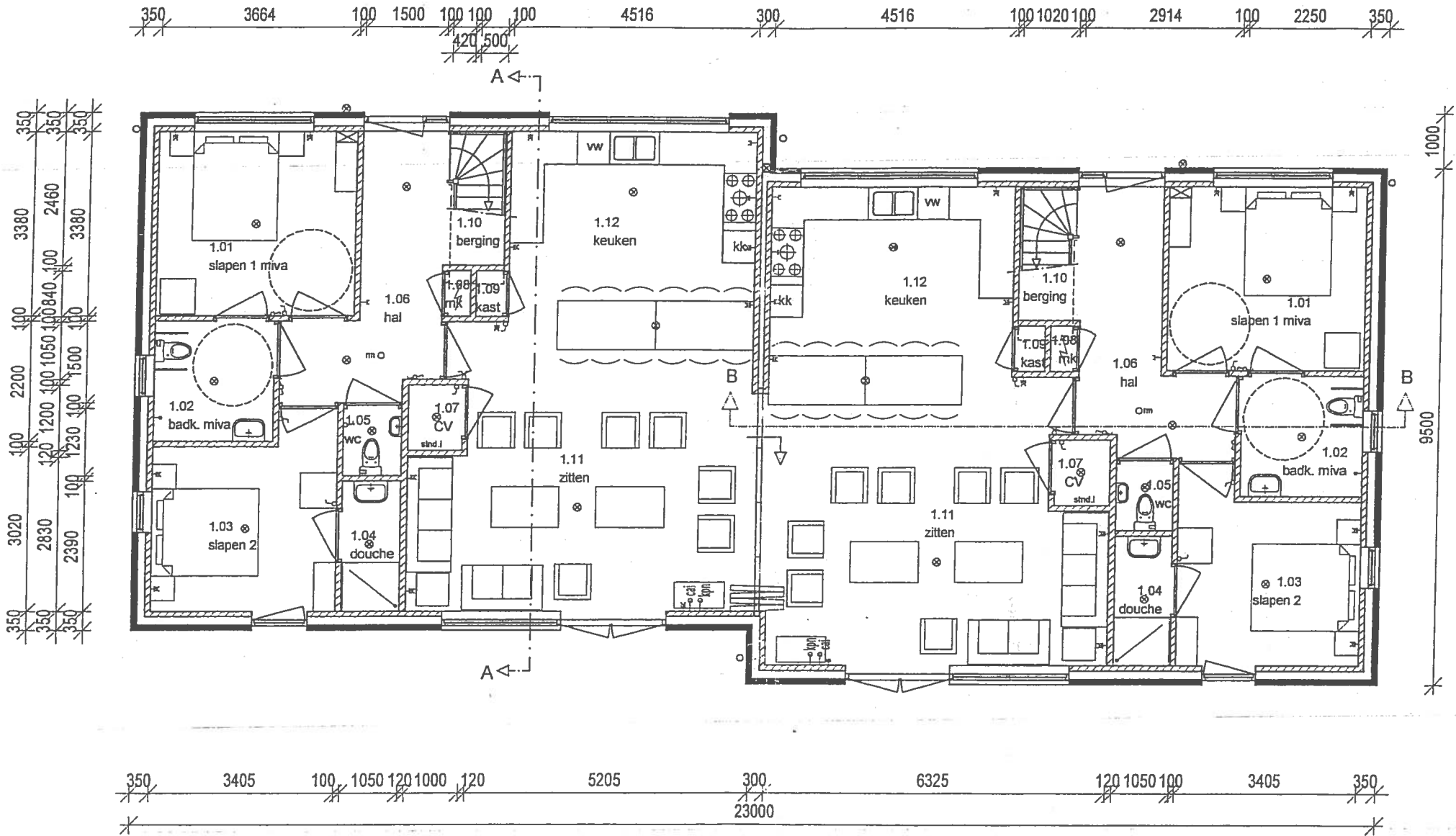
Beganegrond
