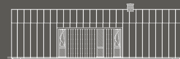
rechter zijgevel
