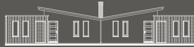
voorgevel
