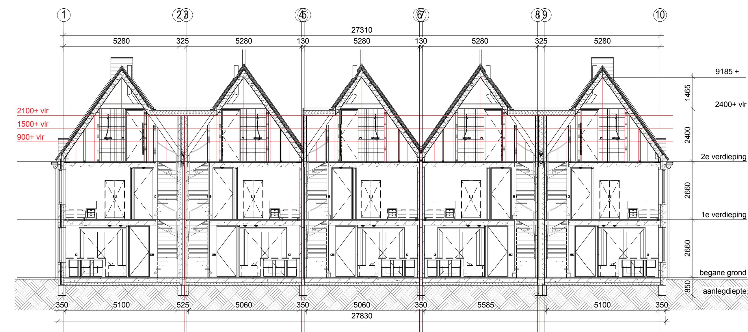
Doorsnede A-A
