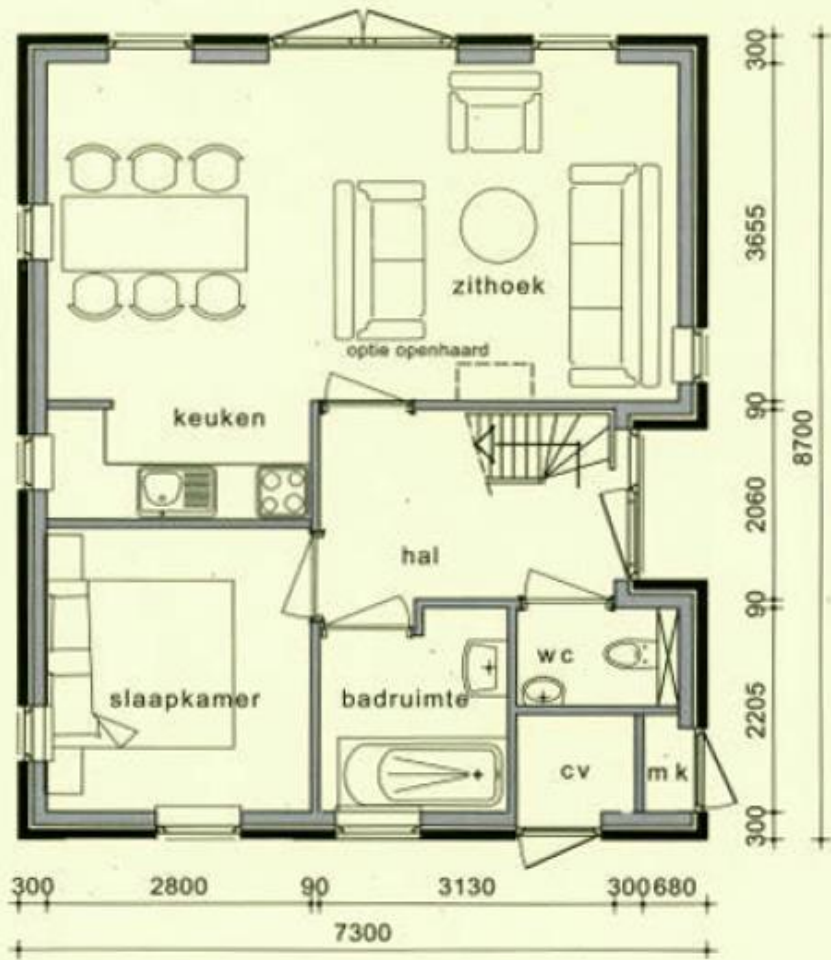
begane grond
