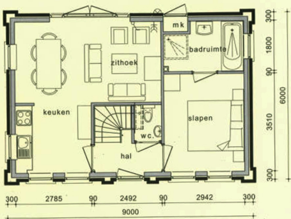
begane grond
