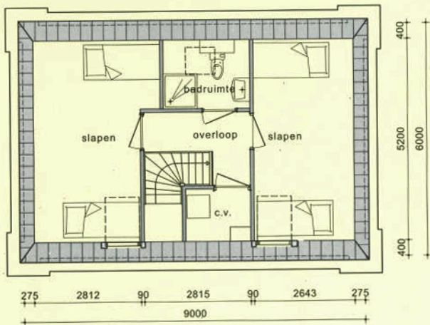
verdieping
